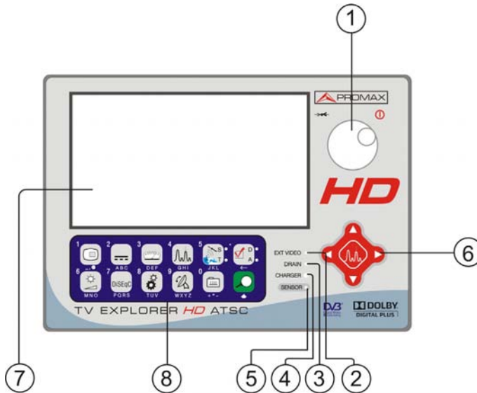
Figura 3.- Panel frontal.
