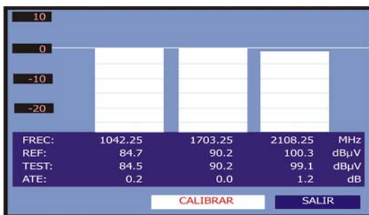
Figura 16.- Prueba FI SAT. Banda Satélite.
