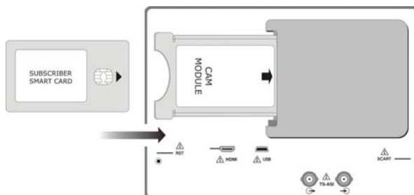
Figure 71.- Insertion d'un module CAM et carte d'abonné (SMART-CARD).
