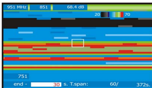
Figura 51.- Représentation du Spectrogramme.
