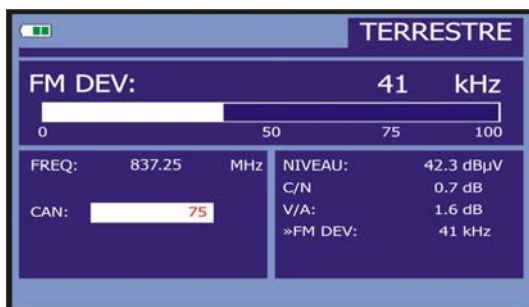
Figure 26.- Mesure de la déviation instantanée de fréquence.
