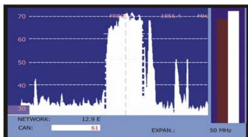
Figure 63.- Outil pour le pointage d'antennes.
