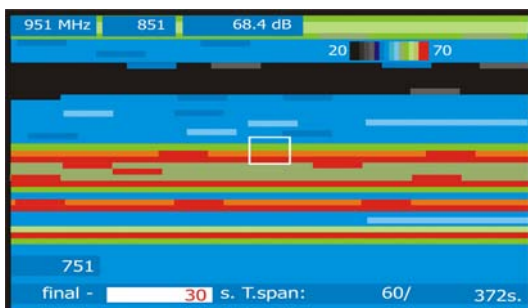
Figura 51.- Representación del espectrograma.
