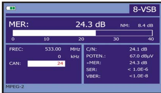
Figura 43.- Pantalla de medida del MER para señales ATSC moduladas en 8-VSB .
