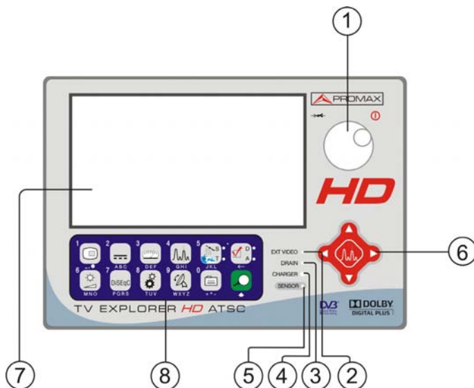
Figure 3.- Panneau frontal.
