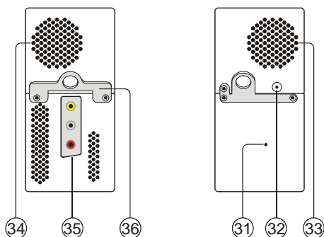
Figure 7.- Eléments du panneau latéral.
