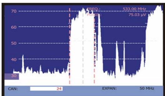
Figure 50.- Mode Analyseur de Spectre.
