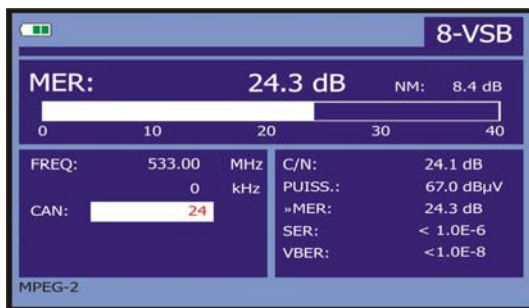
Figure 43- Écran de mesure du MER pour signaux ATSC (8-VSB) .
