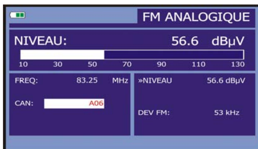
Figure 27.- Mesure du niveau de signal FM Analogique.
