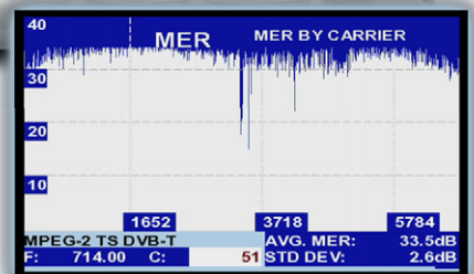
MER por portadora para DVB-T (DVB-T2 opcional)
