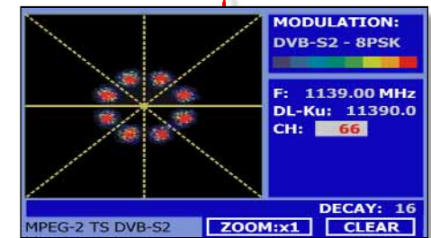
Konstellationsdiagramm
