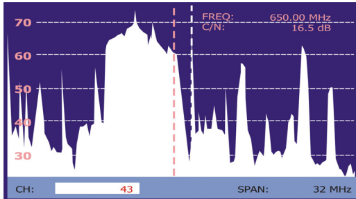
Figure 27.- NOISE cursor. C/N (MANUAL).
